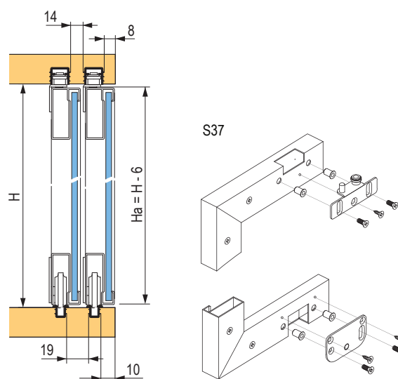
rozměrové schéma pro sadu S37
