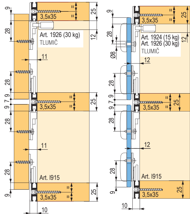
naložená dvířka
