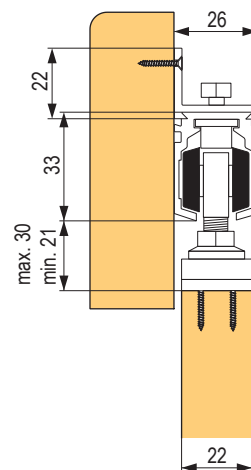
rozměrové schéma – velikost kování a frézování trnu
