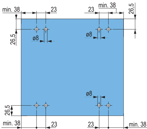
vrtání na vložené skleněné dveře
