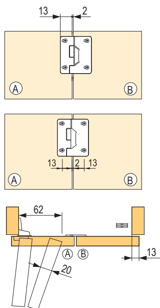
montážní schéma sady bez a se spodním vedením
