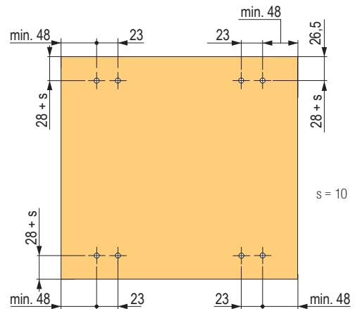
vrtání na naložené dřevěné dveře
