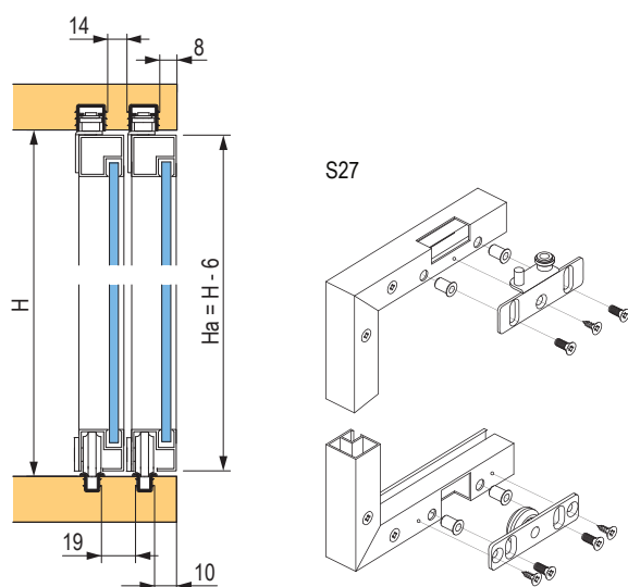
rozměrové schéma pro sadu S27
