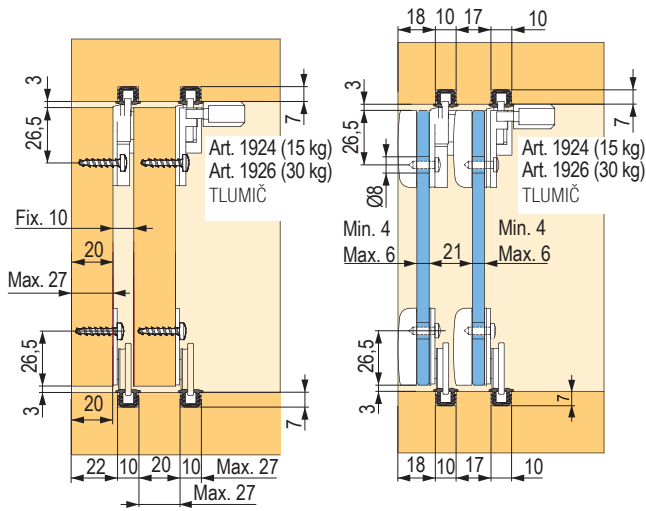
vložená dvířka
