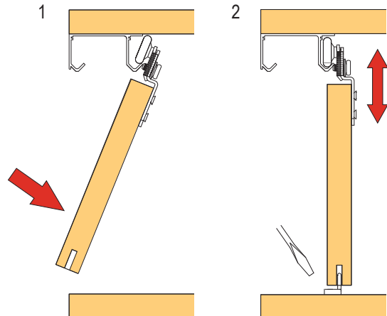
nasazení křídla do profilu a vodícího trnu
