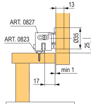
se spodním vedením na dně
