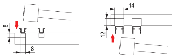
rozměrové schéma pro sadu S37
