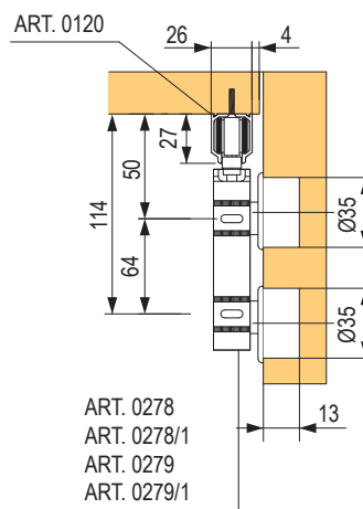
montážní schéma sady pro větší dveře
