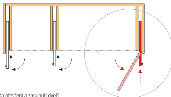
schéma otevření a zasunutí dveří
