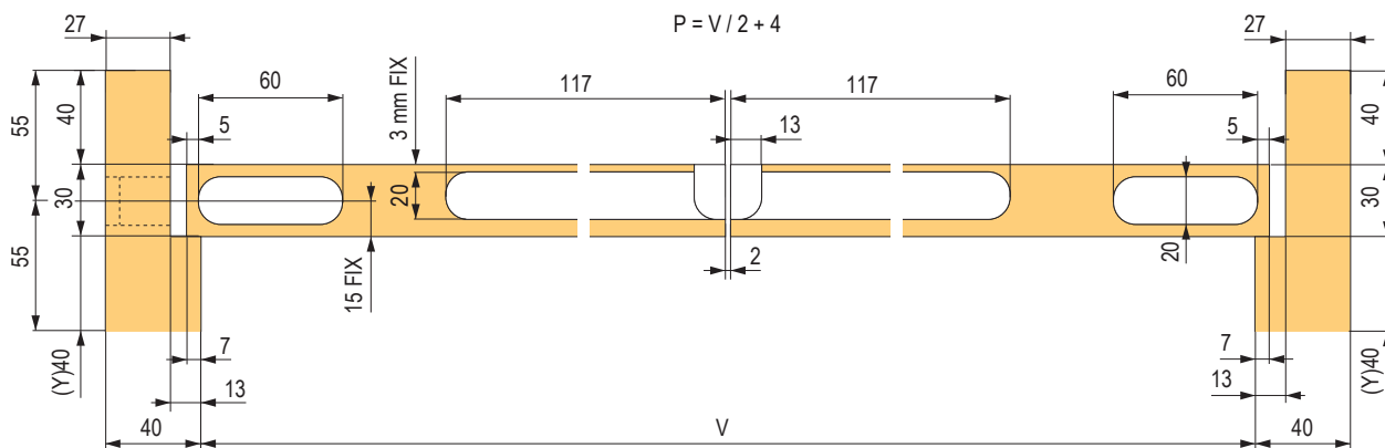
rozměrové schéma
