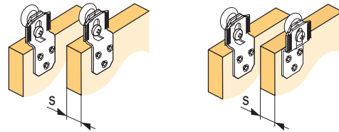
nasazení křídla do profilu a vodícího trnu
