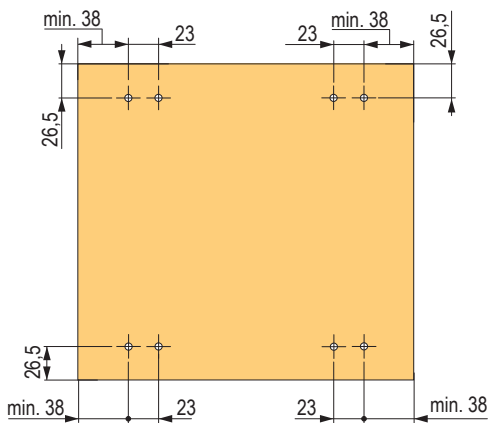
vrtání na vložené dřevěné dveře
