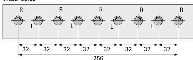
Vrtací obraz
