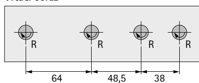
Vrtací obraz
