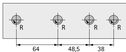
Vrtací obraz
