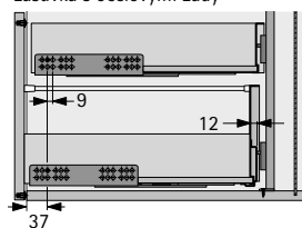
Vnitřní zásuvka a vnitřní vysoká zásuvka s ocelovými zády
