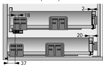
Vnitřní zásuvka a vnitřní vysoká zásuvka s ocelovými zády
