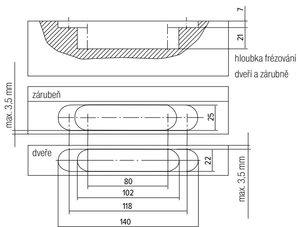
frézování dveří a zárubní pro závěs Symbio 22
