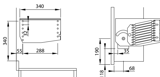
2. Instalace pouzdra do skříně
