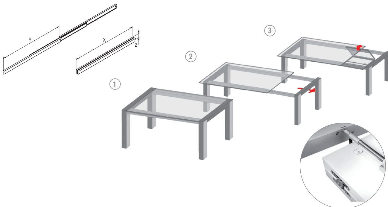
příklad použití překlápěcího systému FM 405122
