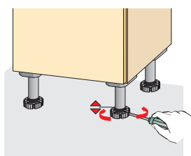
seřízení výšky z čelní strany šroubovákem
