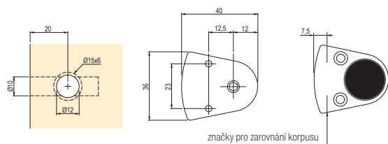
značky pro zarovnání korpusu
