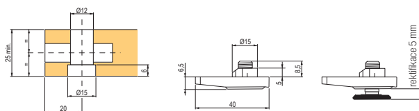
instalace v kombinaci se systémem Target J12
