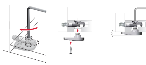
instalace v kombinaci se systémem Target J12
