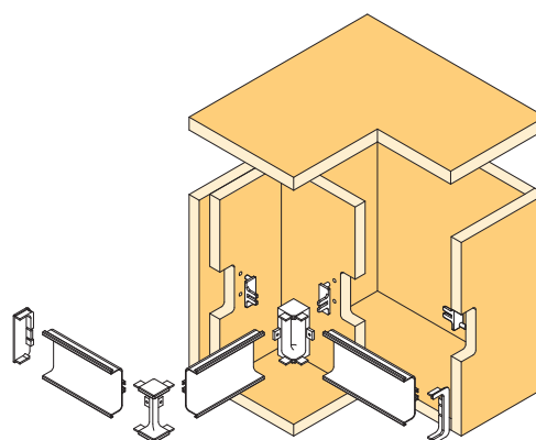
horizontální zásuvkový "C" profil
