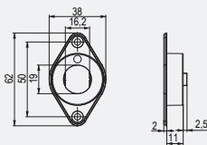
309274 adaptér na montáž do dřeva
