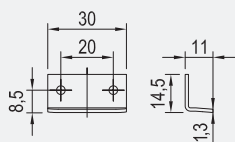
Úhelníková zarážka 30 mm
