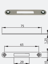
Protikus na zadlabání
