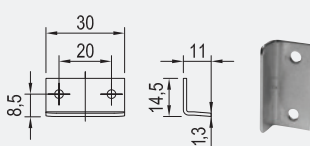
Úhelníková zarážka 30 mm
