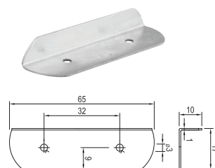
Úhelníková zarážka 65 mm
