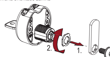
Změna orientace zámku
