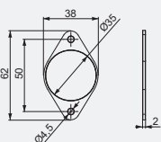
350805 plastová vložka pro montáž do tenkého dřeva, nutno kombinovat s adaptérem 309274
