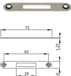
Protikus na zadlabání
