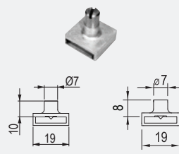
Kolíky k tyči
