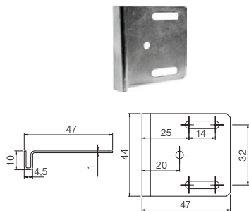
Úhelníková zarážka 44 mm
