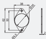
350805 plastová vložka pro montáž do tenkého dřeva, nutno kombinovat s adaptérem 309274
