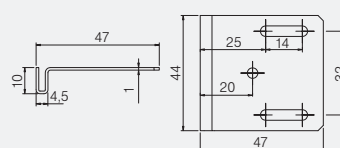
Úhelníková zarážka 44 mm
