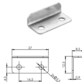
Úhelníková zarážka 27 mm
