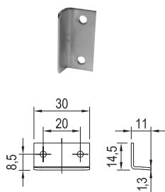
Úhelníková zarážka 30 mm
