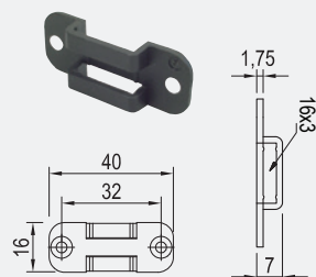
Vodítko tyče
