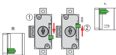
přepínání směru zamykání
