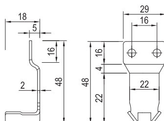
Protikus centrálního zámku pro kolečkové výsuvy s bočnicí (metabox)
