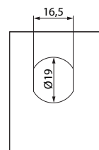
vrtání otvoru
