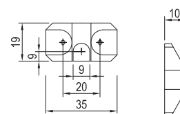
Protikus centrálního zámku pro dřevěnou zásuvku
