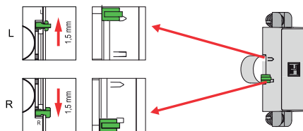
aktivace blokace klíče (u odemknutého zámku nelze vytáhnout klíč)
