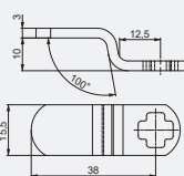
309277 závora 400 zakřivená
