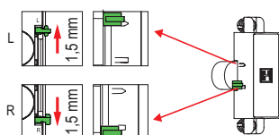
aktivace blokace klíče (u odemknutého zámku nelze vytáhnout klíč)
