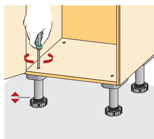
seřízení výšky shora šroubovákem
