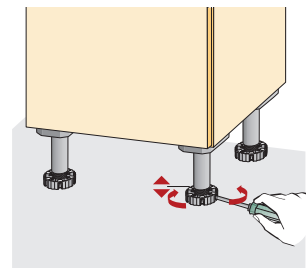
seřízení výšky z čelní strany šroubovákem
