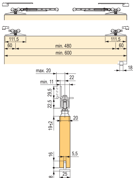
dveřní kování pro 30 kg (brzda, kapalinový tlumič)
