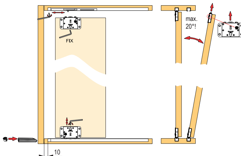
nasazení křídla a nastavení
