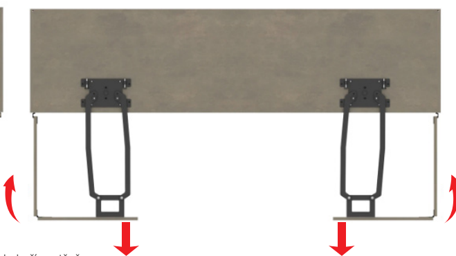
příklad vložených dveří ve stěně
