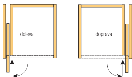
příklad otevírání skládaných dveří Concepta III Push 1× levé dveře Concepta III Push 1× pravé dveře
