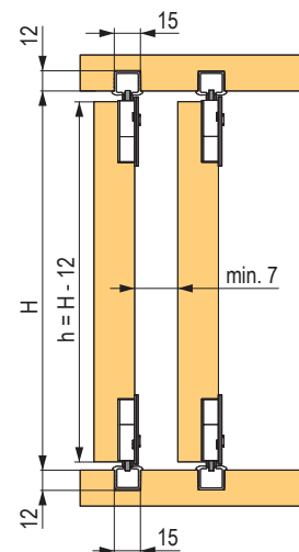
otvor pro spodní vozík
