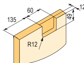
otvor pro horní vozík
