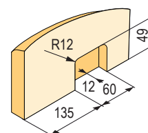
otvor pro spodní vozík
