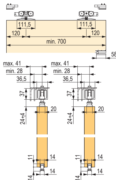
dveřní kování pro 160 kg (brzda)
