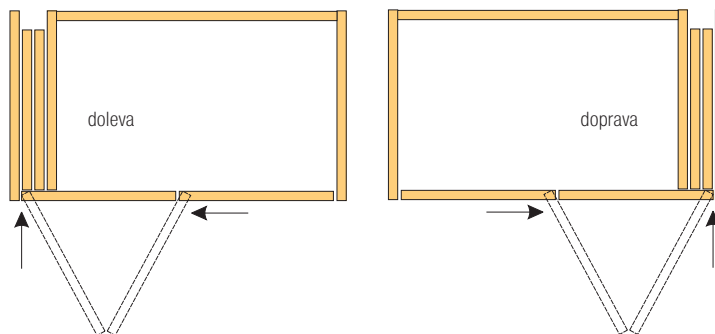
příklad otevírání skládaných dveří Concepta III Push 1× levé dveře + Folding Concepta III Push 2× pravé dveře
