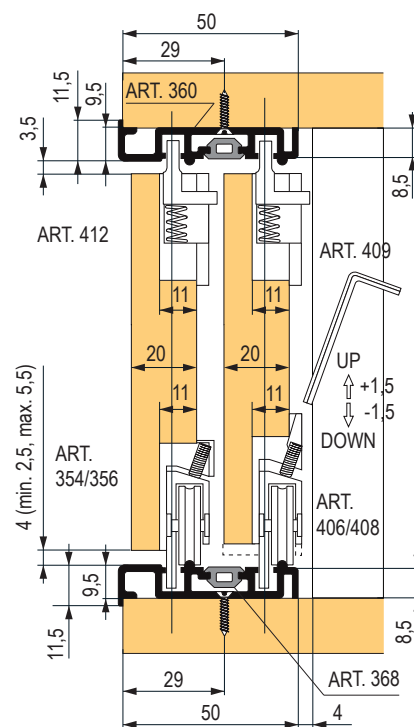
rozměrové schéma – dvojitý profil
