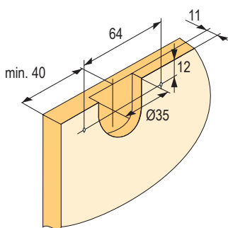
otvor pro horní vozík
