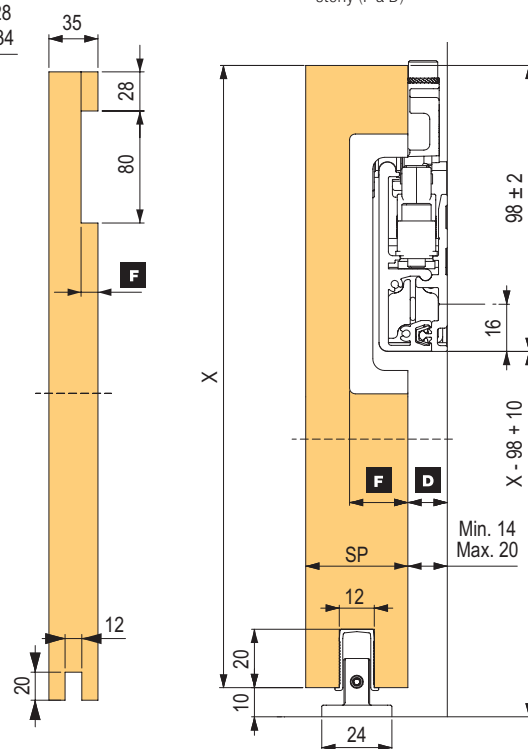
hloubkou frézování ovlivníte odsazení křídla od stěny (F a D)
