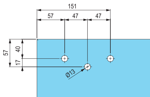
vrtání skla pro upevnění vozíku
