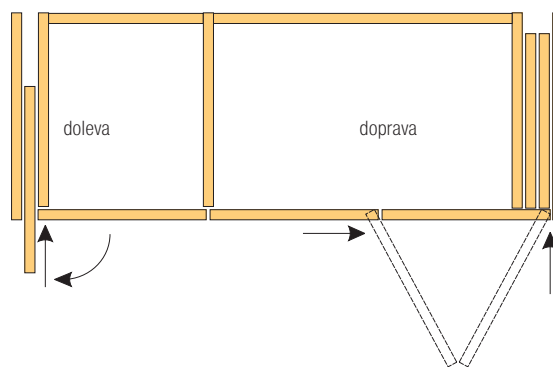
příklad otevírání skládaných dvířek Folding Concepta III Push 2× levé dveře a 2× pravé dveře
