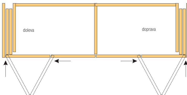
příklad otevírání skládaných dvířek Folding Concepta III Push 2× levé dveře a 2× pravé dveře
