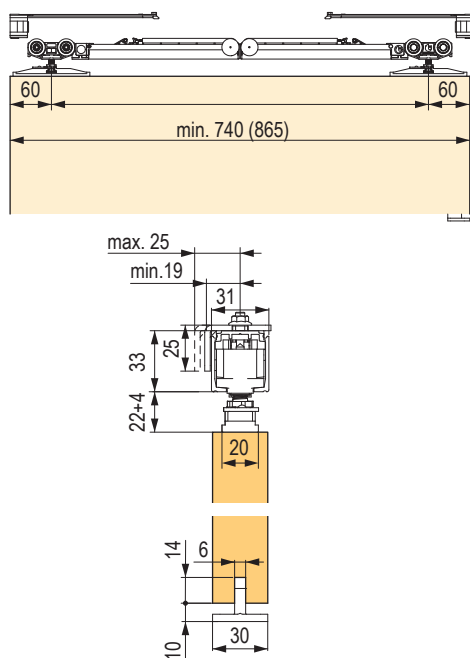
dveřní kování pro 50–160 kg (kapalinový tlumič)
