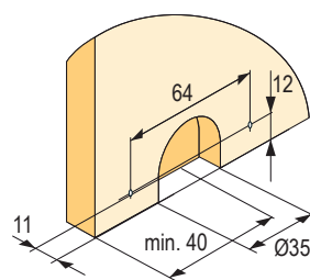
otvor pro horní vozík
