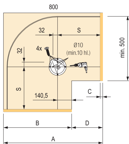
montáž nosné tyče, korpus 800 mm
