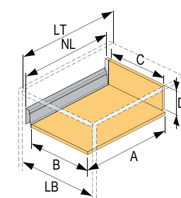
Čelní zásuvka, výška 70/144 mm
