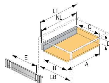
Vnitřní zásuvka, výška 70 mm
