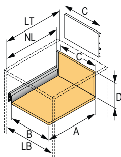
Vnitřní zásuvka, výška 94 a 126/282 mm
