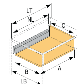
Čelní zásuvka, výška 70/176 mm
