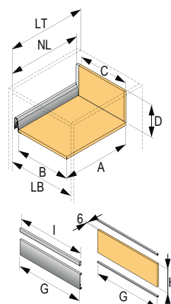
Vnitřní zásuvka, výška 94 a 126/218 mm
