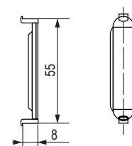
509772 PLASTOVÁ MISKA MĚLKÁ k protiplechu pro bezfalcové dveře
