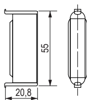
509768 PLASTOVÁ MISKA HLUBOKÁ k protiplechu pro bezfalcové dveře
