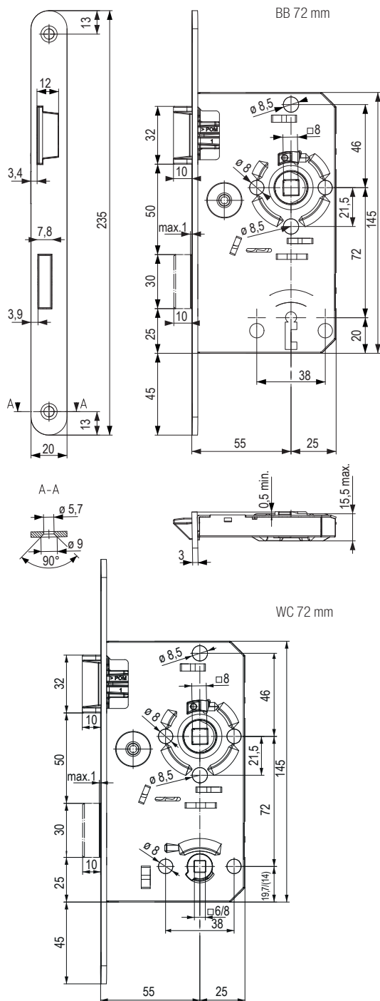
plastová střelka závora BB/72 mm
