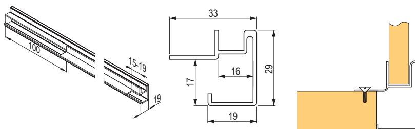
Nákres krácení vodicí lišty
