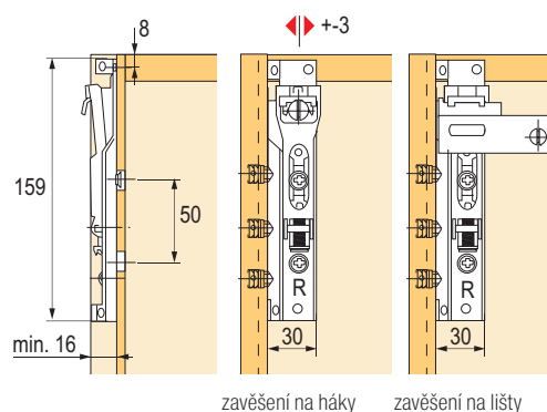
zavěšení na háky
