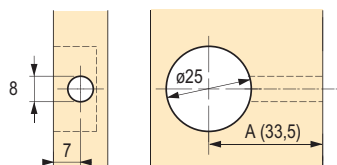
schéma vrtání
