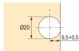
schéma vrtání dílce
