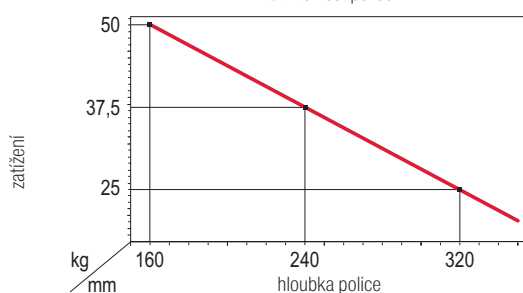
zátěžnost police
