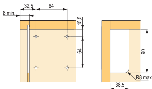
vrtačí plán s použitím krytky
