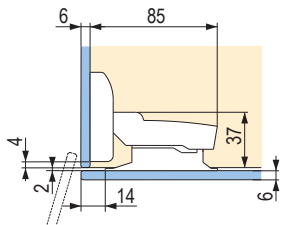
Naložené dveře s mezerou 2 mm
