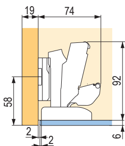
Vložené dveře
