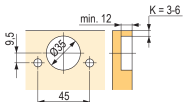
Vrtání závěsů TB
