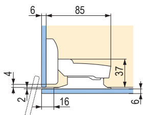
Zcela naložené dveře (bez mezer)
