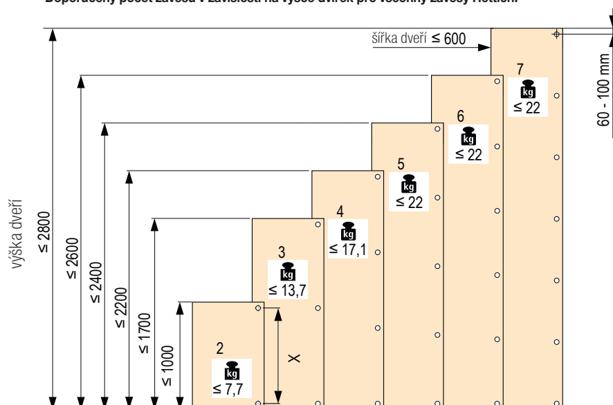
Doporučený počet závěsů v závislosti na výšce dveří pro všechny závěsy Hettich.
