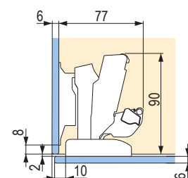
Naložené dveře s mezerou 2 mm
