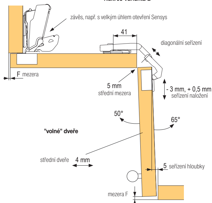
Nákres Varianta B
