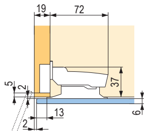
Naložené dveře s mezerou 2 mm
