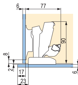
Naložené dveře s přesahem dveří 11 mm
