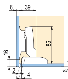
Vložené dveře s mezerou 2 mm
