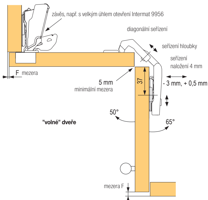
Nákres Varianta A
