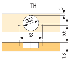
Vrtání závěsů TH
