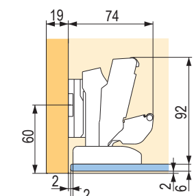
Vložené dveře s odsazením 2 mm
