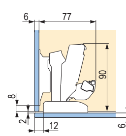
Zcela naložené dveře (bez mezer)
