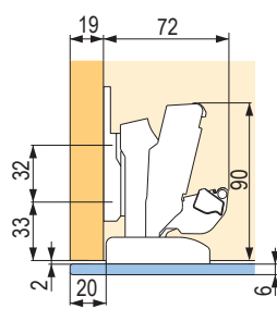
Zcela naložené dveře (bez mezer)
