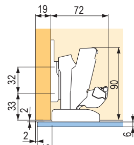
Naložené dveře s mezerou 2 mm
