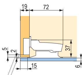
Zcela naložené dveře (bez mezer)
