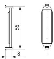
509772 CUVETTE PLASTIQUE PEU PROFONDE pour gâche pour porte sans feuillure
