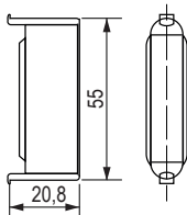
509768 CUVETTE PLASTIQUE PROFONDE pour gâche pour porte sans feuillure
