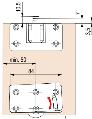
Umístění a rozměr vozíků
