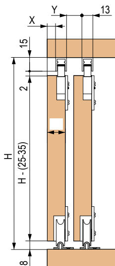
Rozměrové schéma
