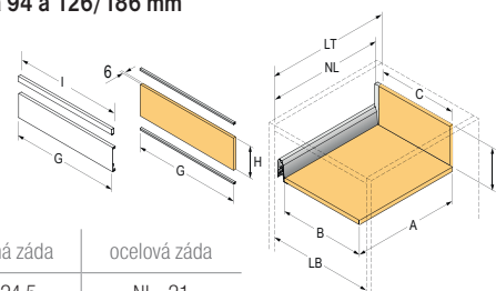
Vnitřní zásuvka, výška 94 a 126/186 mm
