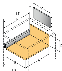
Čelní zásuvka, výška 94 a 126/186 mm
