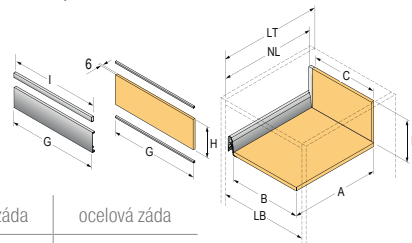
Vnitřní zásuvka, výška 94 a 126/218 mm
