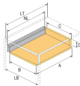
Čelní zásuvka, výška 54 mm
