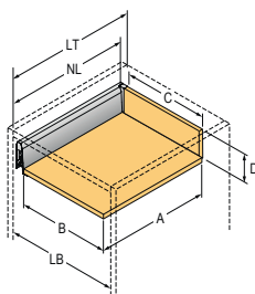
Vnitřní zásuvka, výška 126 mm
