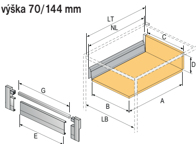
Vnitřní zásuvka, výška 70/144 mm
