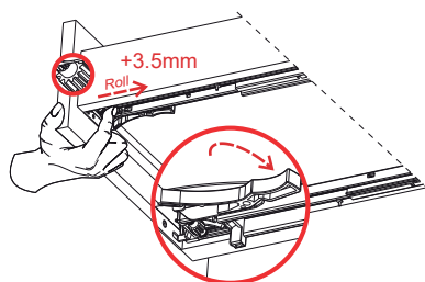
vysazení zásuvky
