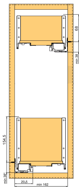
LEGRABOX
