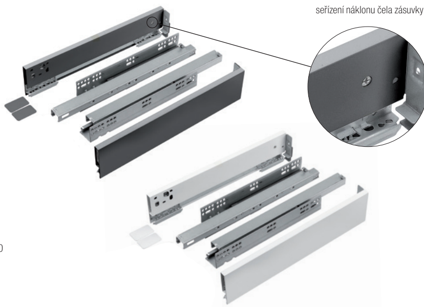
seřízení náklonu čela zásuvky
