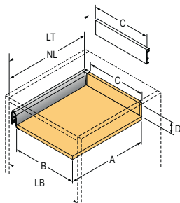
Vnitřní zásuvka, výška 94 mm
