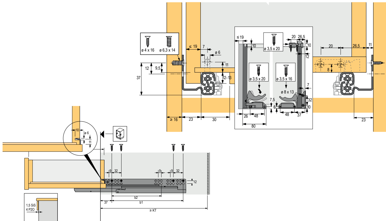
Celovýsuv Quadro V6
