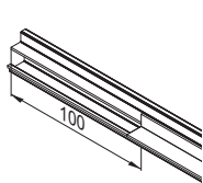
Nákres krácení vodící lišty
