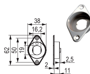
309274 adaptér na montáž do dřeva
