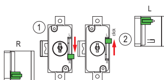
přepínání směru zamykání
