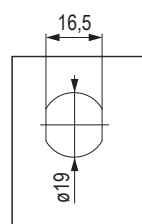
vrtání otvoru do plechových dveří
