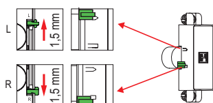
aktivace blokad klíče (u odemknutého zámku nelze vytáhnout klíč)
