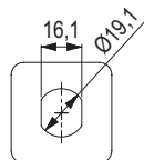
vrtání otvoru do plechových dveří
