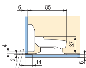
Naložené dveře s mezerou 2 mm
