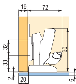
Zcela naložené dveře (bez mezery)
