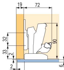
Naložené dveře s mezerou 2 mm
