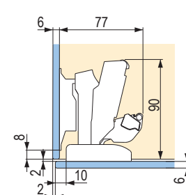
Naložené dveře s mezerou 2 mm
