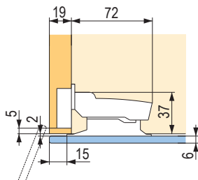
Zcela naložené dveře (bez mezery)
