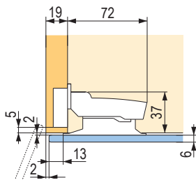
Naložené dveře s mezerou 2 mm
