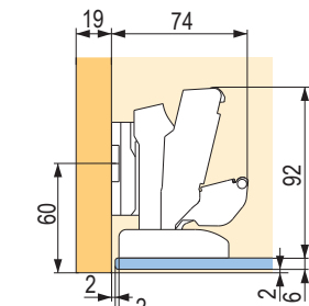
Vložené dveře s odsazením 2 mm
