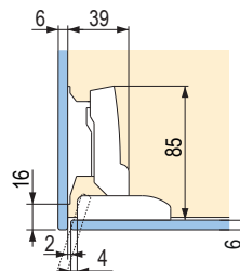
Vložené dveře s mezerou 2 mm
