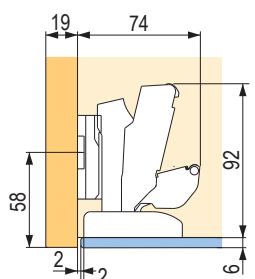
Vložené dveře
