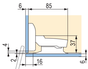
Zcela naložené dveře (bez mezery)
