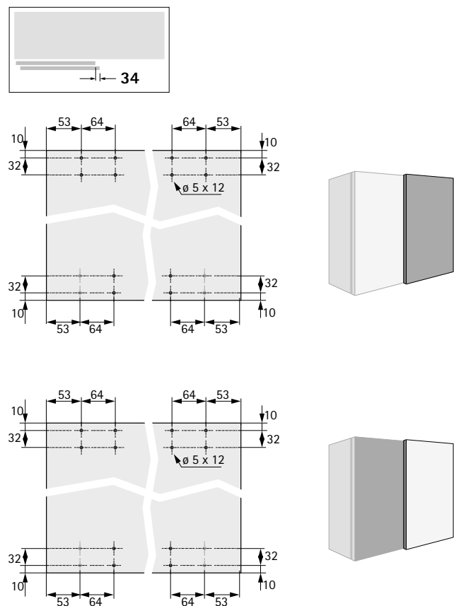
Vrtací obraz - přesazení dveří 34 mm
