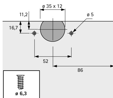
Adaptér pro dřevěné dveře k přišroubování
