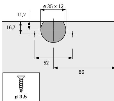
Adaptér pro dřevěné dveře k přišroubování
