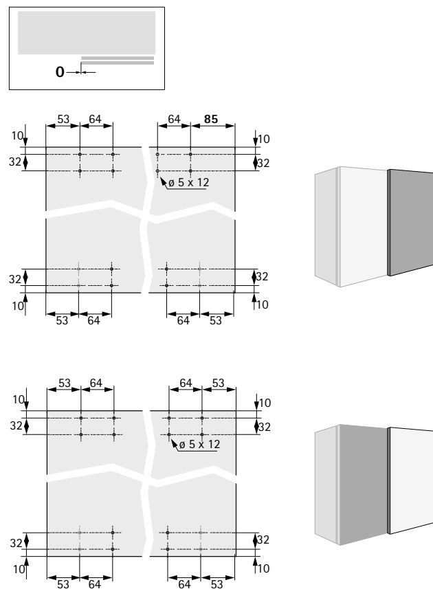
Vrtací obraz - přesazení dveří 0 mm
