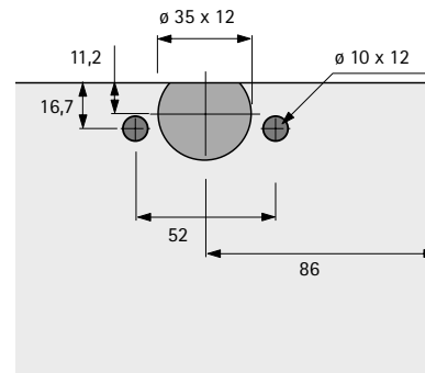
Adaptér pro dřevěné dveře k zalisování
