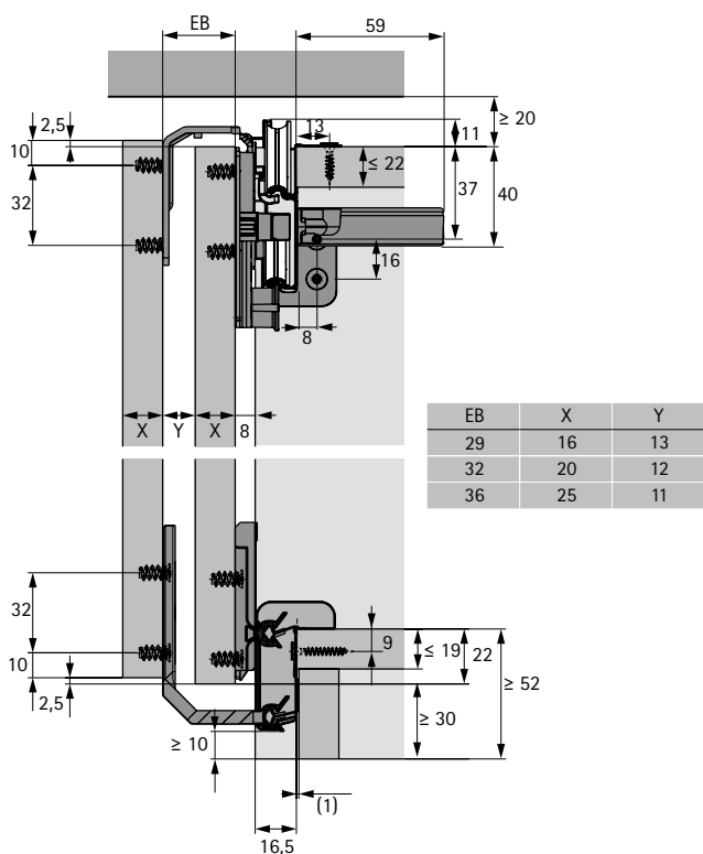
Vrtací obraz - přesazení dveří 34 mm
