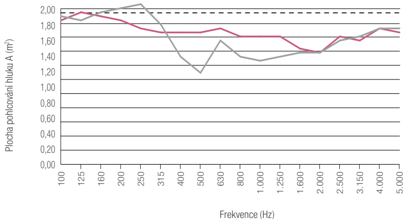
Ekvivalentní plocha pohlcování hluku podle ISO 354 (dozvuková komora) – skříně s čelní plochou 1,91 m 2
